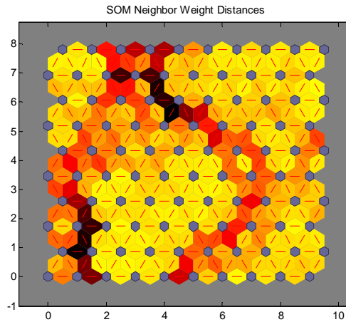
Figure 4. SOM Neighbour Distances
