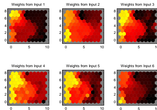
Figure 5. SOM Weight Planes
